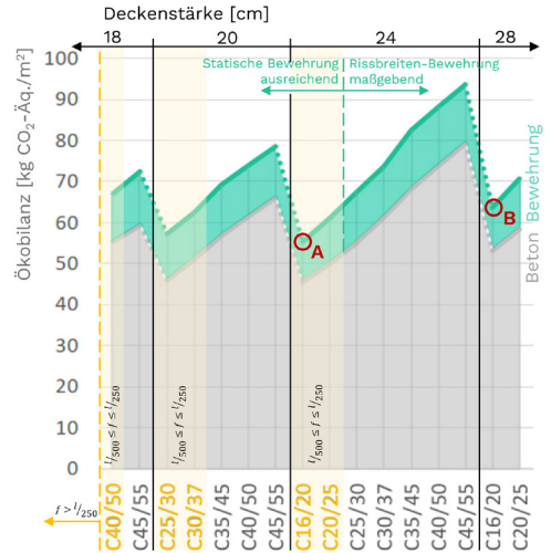
Ökobilanz für einachsige, 6m spannende Betondecke
