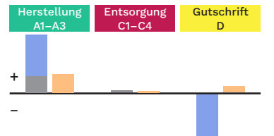
Primärstahl prozessbedingt energiebedingt Sekundärstahl energiebedingt Qualitative CO 2 -Emissionen im Lebenszyklus (Abb. 3.8)
